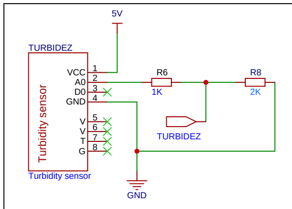
SENSOR DE TURBIDEZ
