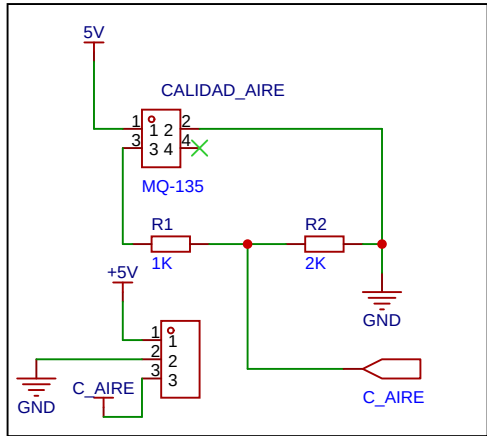
SENSOR DE CALIDAD DEL AIRE
