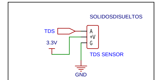
SENSOR DE SÓLIDOS DISUELTOS
