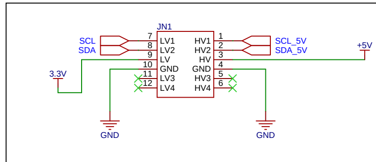
CONVERTIDOR DE NIVEL LÓGICO 12C
