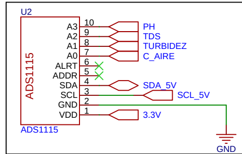
CONVERTIDOR ANALÓGICO DIGITAL
