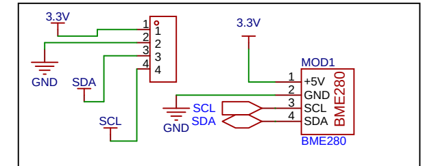
SENSOR DE PRESIÓN, TEMPERATURA Y HUMEDAD
