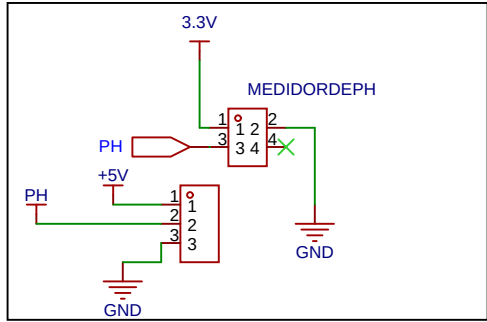
MEDIDOR DE PH
